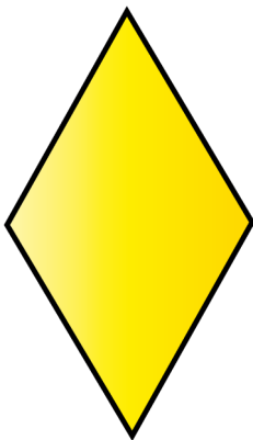
rhombus
