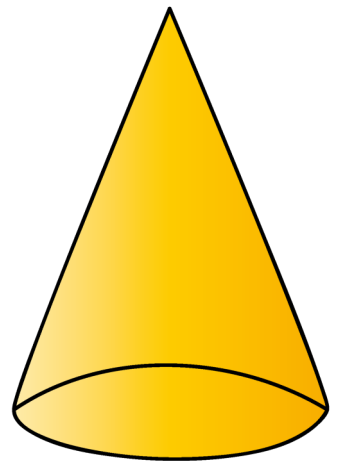
cone
